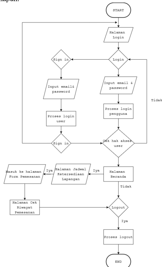
Gambar 5. Flowchart Pengguna
