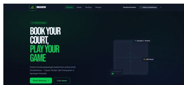
Gambar 8. Halaman Beranda
