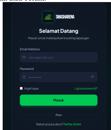
Gambar 12. Halaman Login
