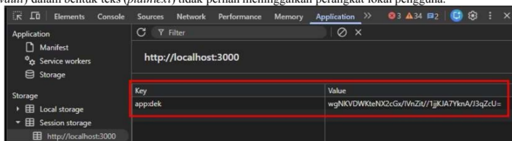
Gambar 5. Penyimpanan DEK pada Session Storage
