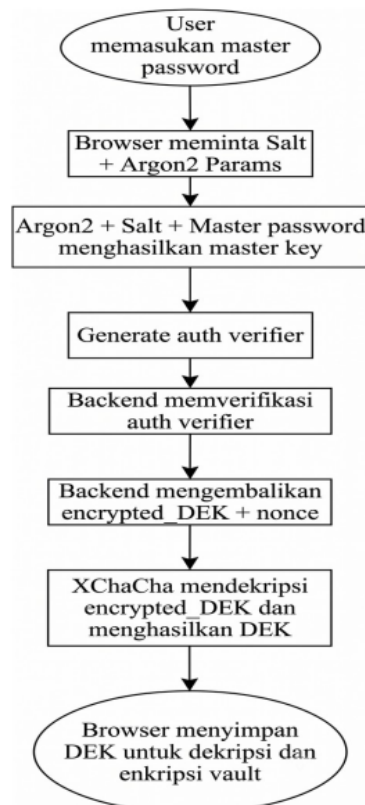
Gambar 2. Arsitektur Enkripsi
