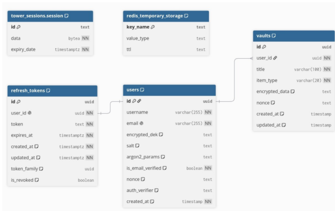
Gambar 3. Perancangan Basis Data
