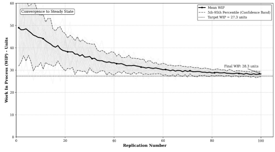
Gambar 7. Grafik Konvergensi WIP
