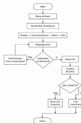
Gambar 1. Flowchart Sistem Media Pembelajaran
