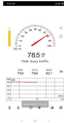
Gambar RPM 4500 Knalpot Standart
