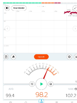
Gambar RPM 4500 knalpot racing dengan DB Killer Aluminium
