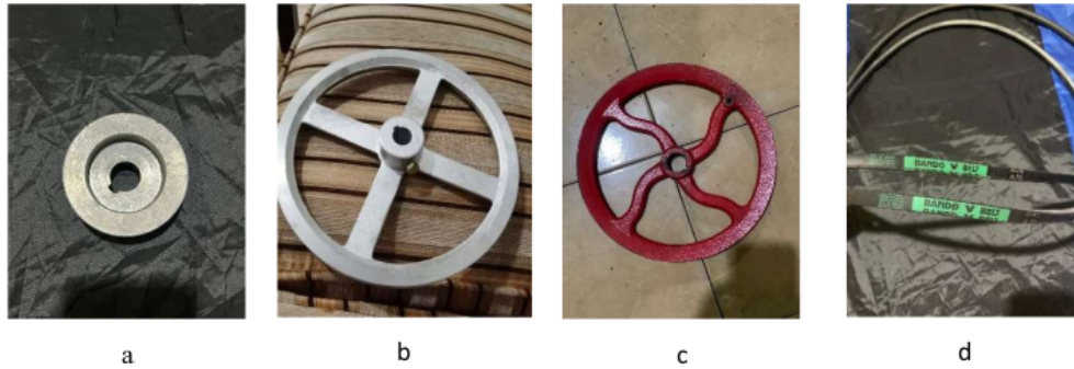
Gambar 3 Perangkat Transmisi
