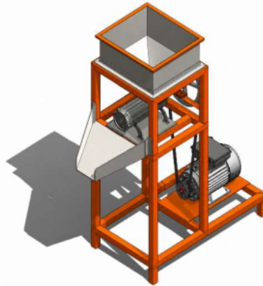
Gambar 2 Desain mesin pencetak pellet
