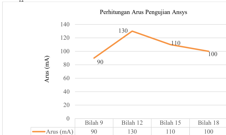
Gambar 8. Grafik Perhitungan Arus
