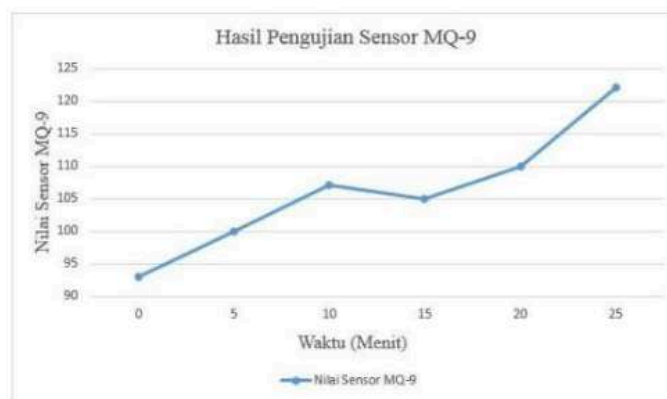
Gambar 7. Grafik Hasil Pengujian Sensor MQ-9
