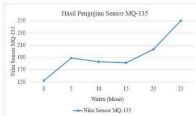
Gambar 8. Garfik Hasil Pengujian Sensor MQ-135
