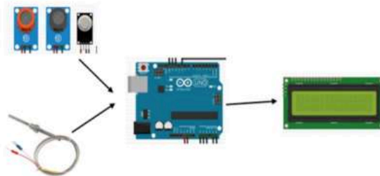
Gambar 4. Perancangan Alat
