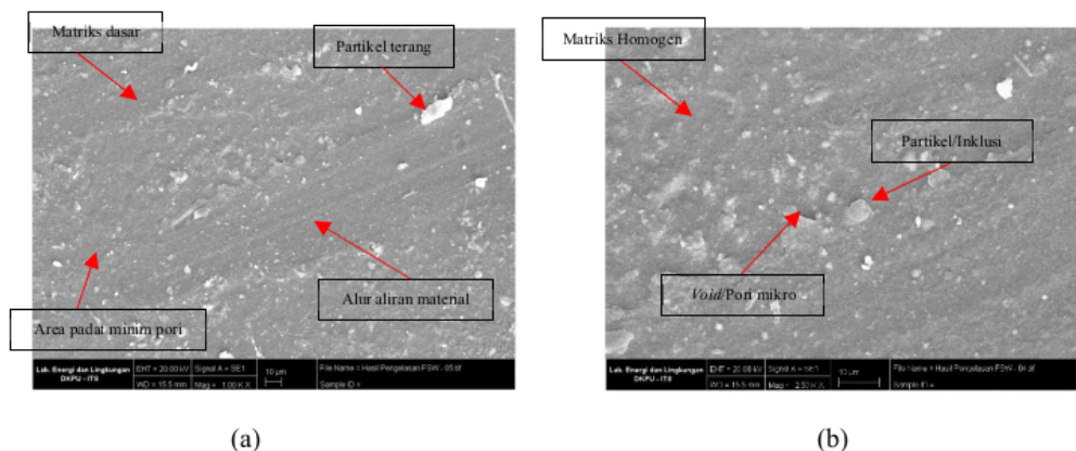
Gambar 12 (a) Uji SEM SP9, (b) Uji SEM sampel tanpa pemanas (STP)
