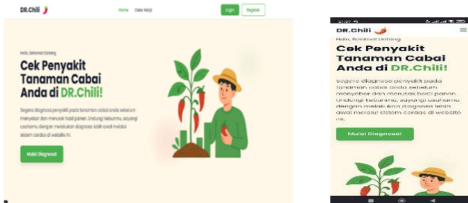
Gambar 6 Halaman Beranda
