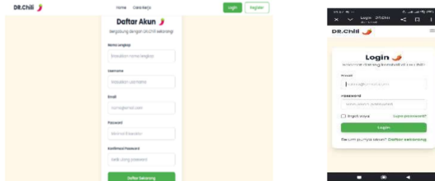
Gambar 7 Halaman login
