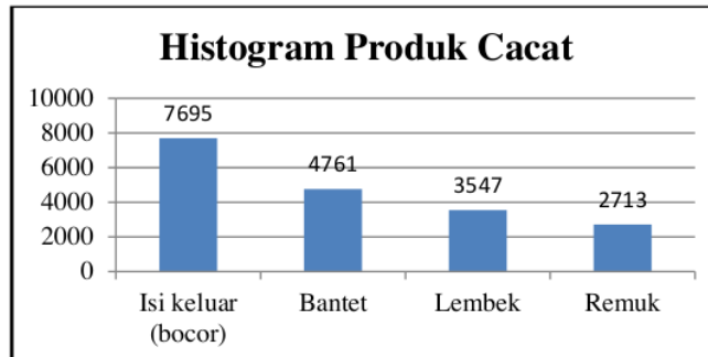
Gambar 1 Histogram Defect Produk Februari-Maret 2022
