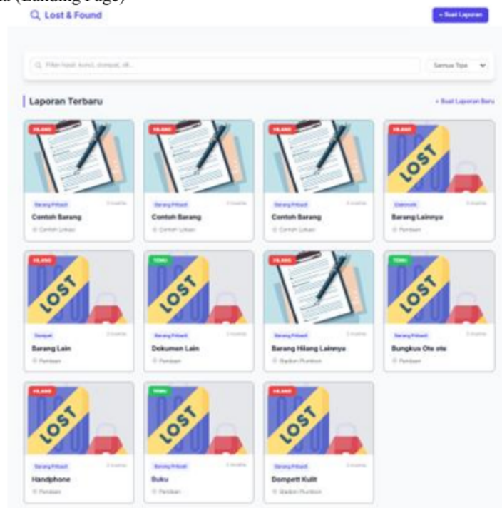
Gambar 6. Halaman utama
