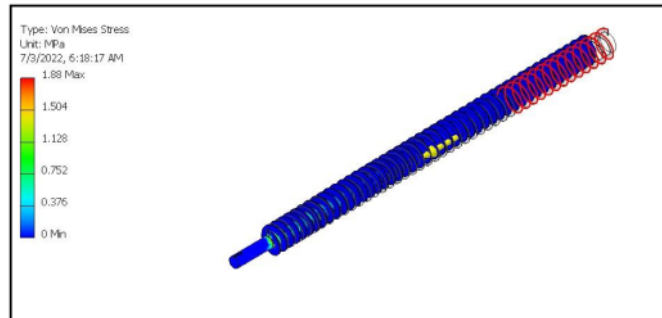
Gambar 5. Deformasi ketika diberi pembebanan
