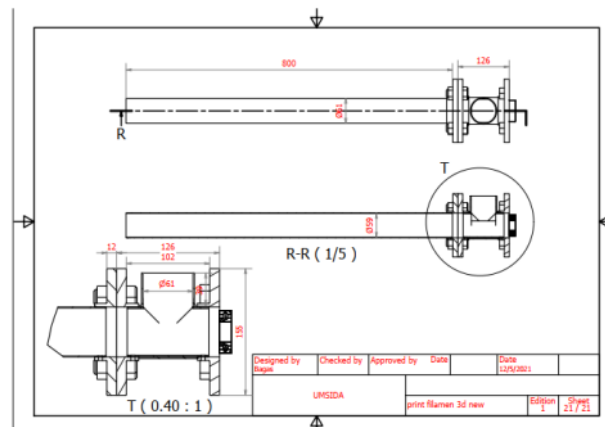
Gambar 6. Desain Barrel dan Letak Thermal Barrier
