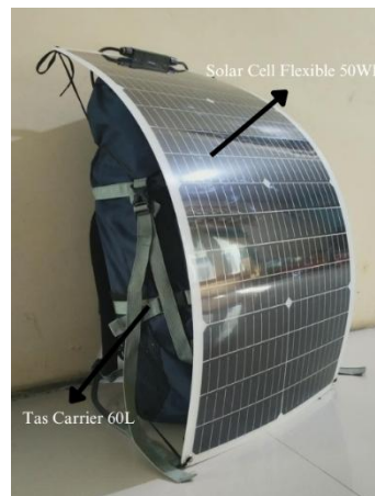
Gambar 4. Tampak Luar Prototipe Panel Surya Untuk Pendakian
