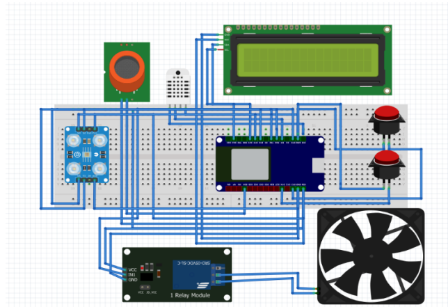
Gambar 3 Perancangan Elektronika Alat Pendeteksi Kesegaran Ikan
