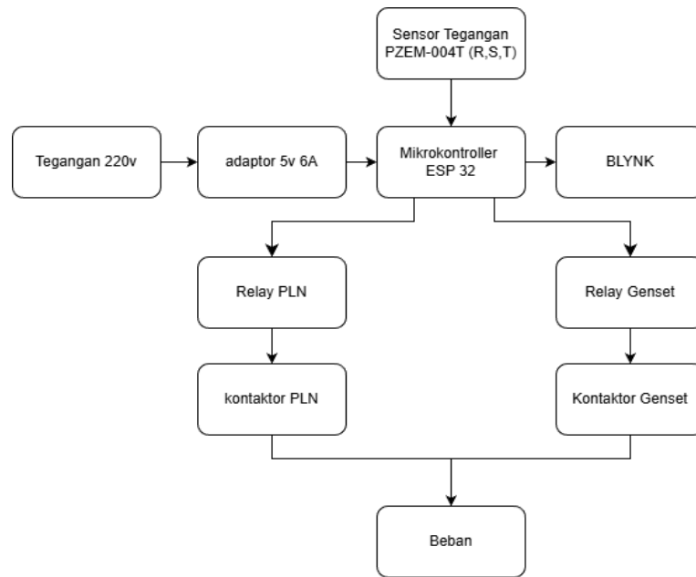
Gambar 2. Blok Diagram Sistem Sekarang.
