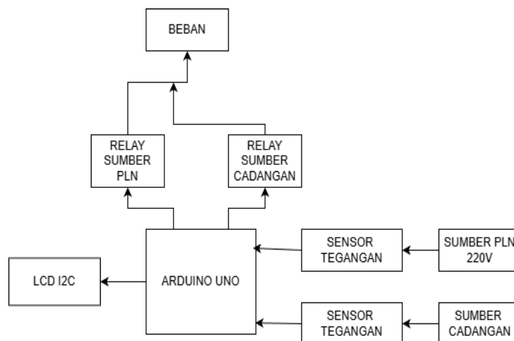
Gambar 1. Blok Diagram Sistem Terdahulu
