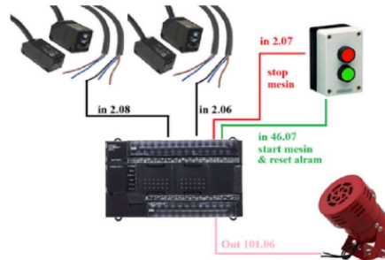
Gambar 4. Rangkaian Perangkat Keras
