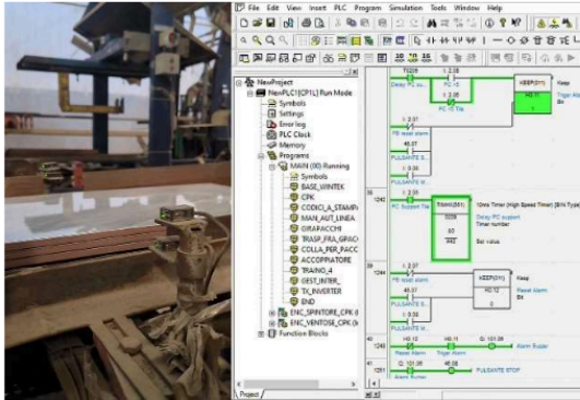
Gambar 9. Pengujian Saat jumlah keramik kurang dari 5
