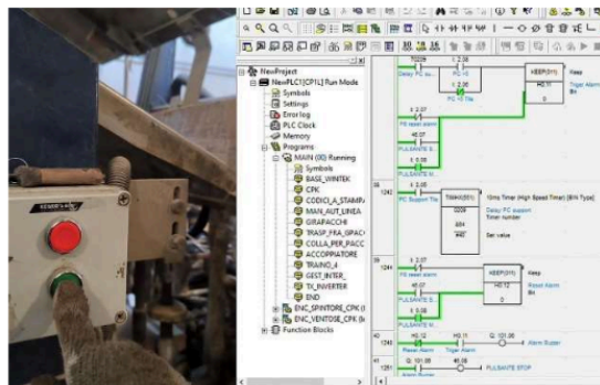
Gambar 8. Pengujian Saat Reset buzzer dan menjalankan mesin kembali
