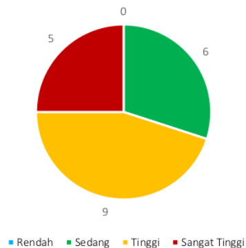
Gambar 1. Kategori Risiko
