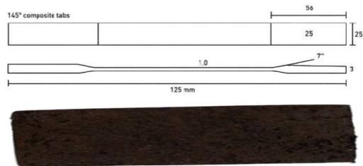
Gambar 4. Bentuk Spesimen Uji Tarik
