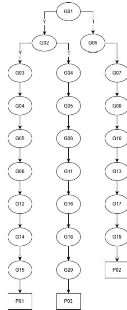
Gambar 2.1 Pohon Keputusan
