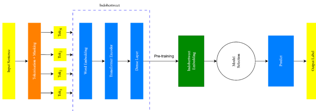
Gambar 2. IndoBERTweet Layer
