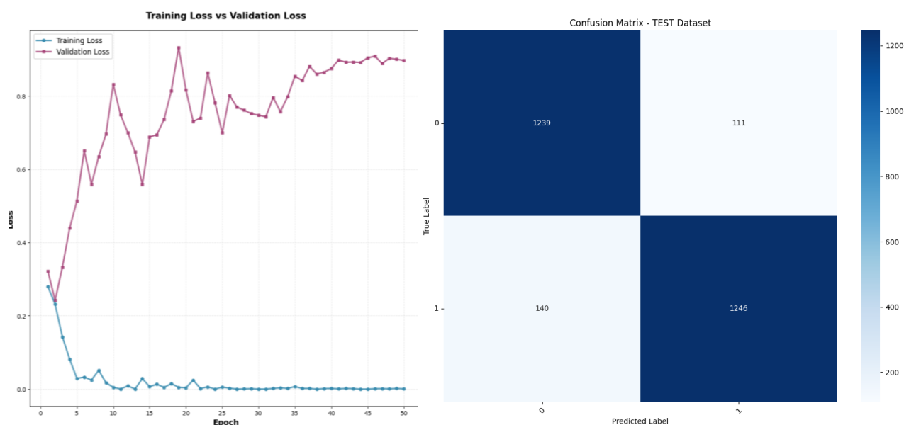
Gambar 4. Training, Validation Loss dan Confusion Matrix Skenario Kedua
